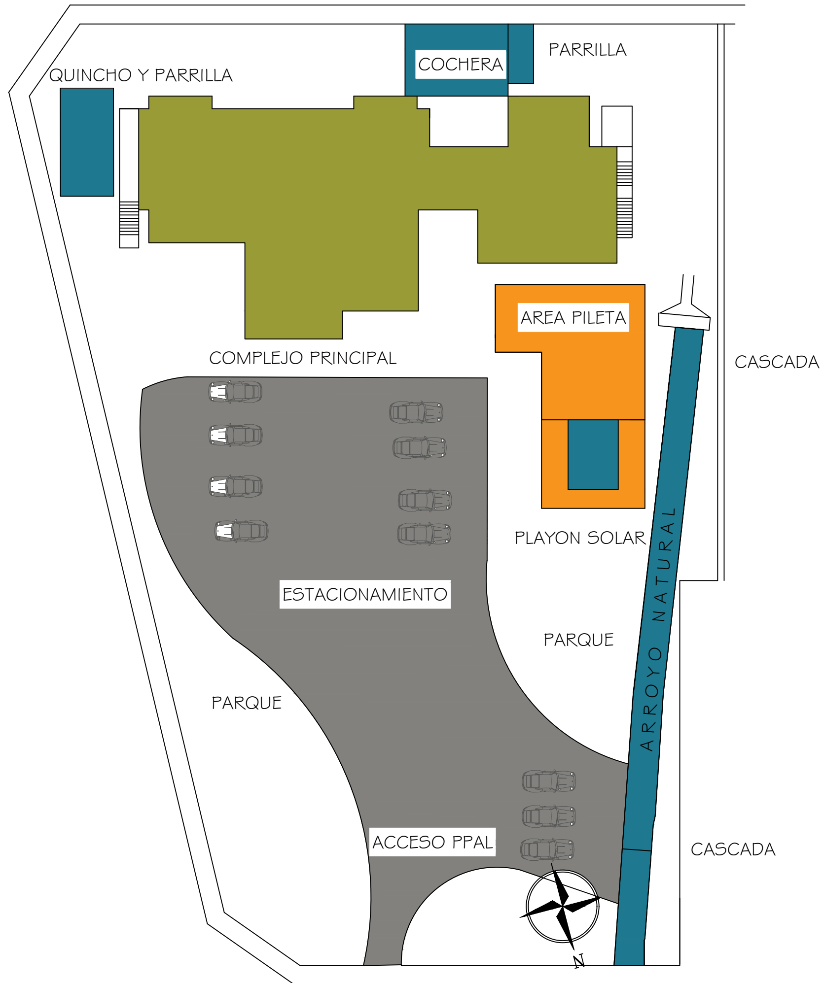
IMPLANTACION DE CONJUNTO
